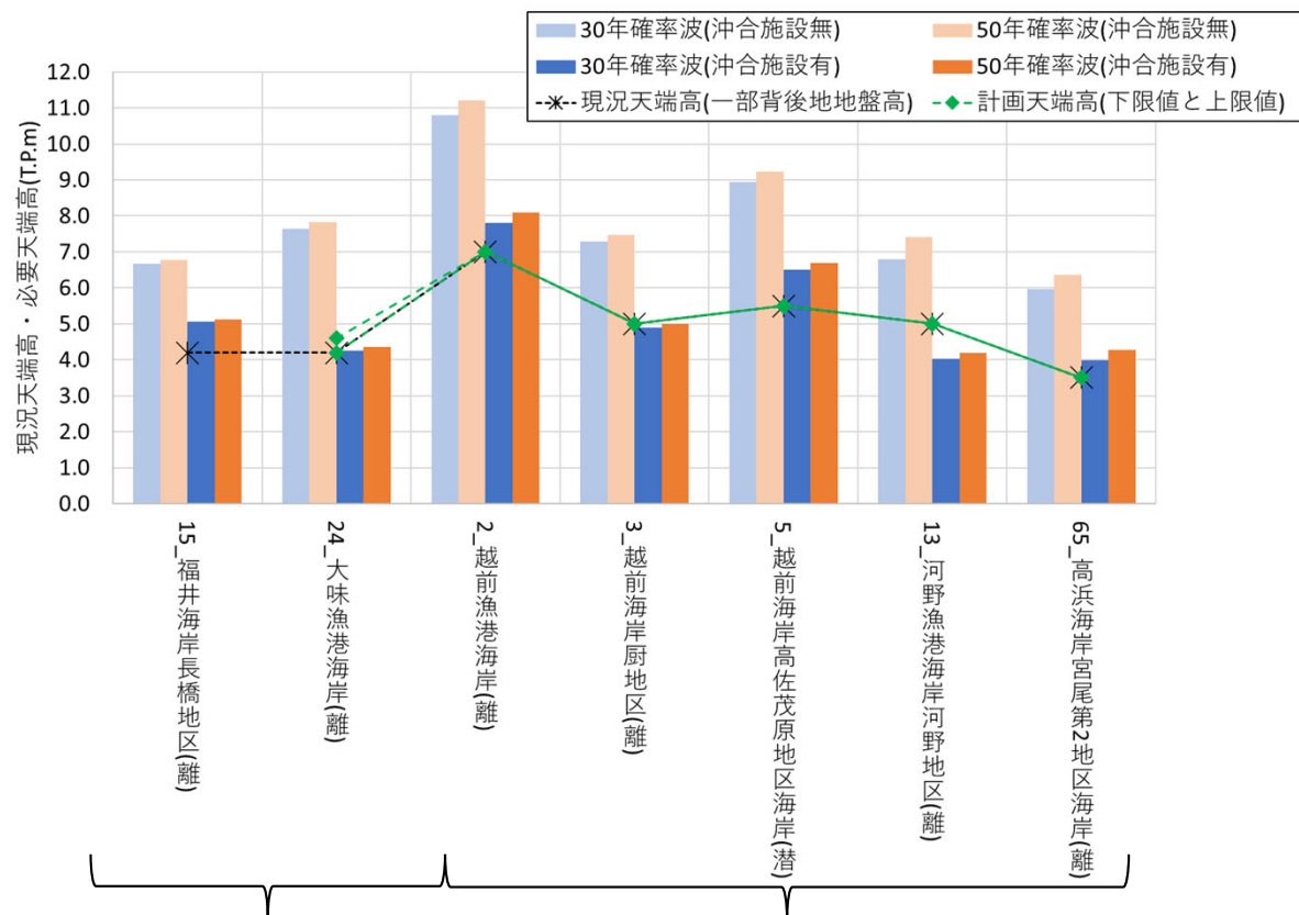
沖合施設を考慮した場合の必要天端高
