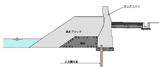
護岸断面図
