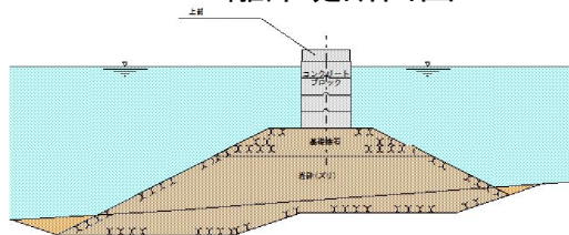
離岸堤断面図
