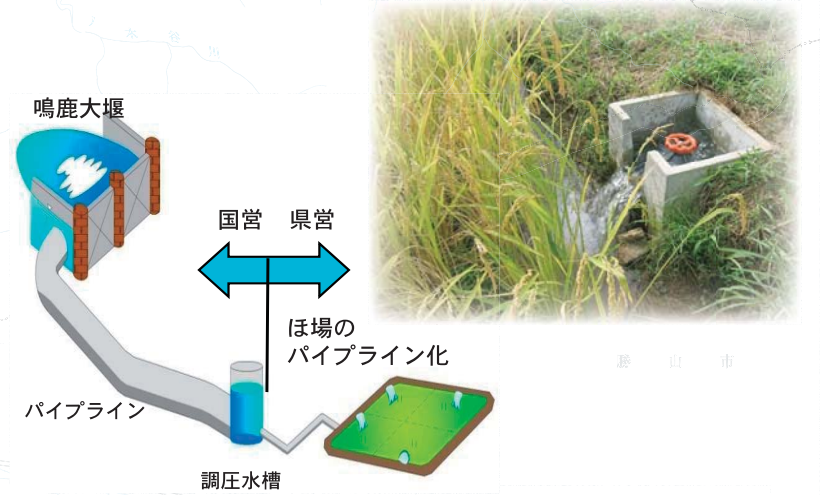
自然圧パイプラインのイメージ
