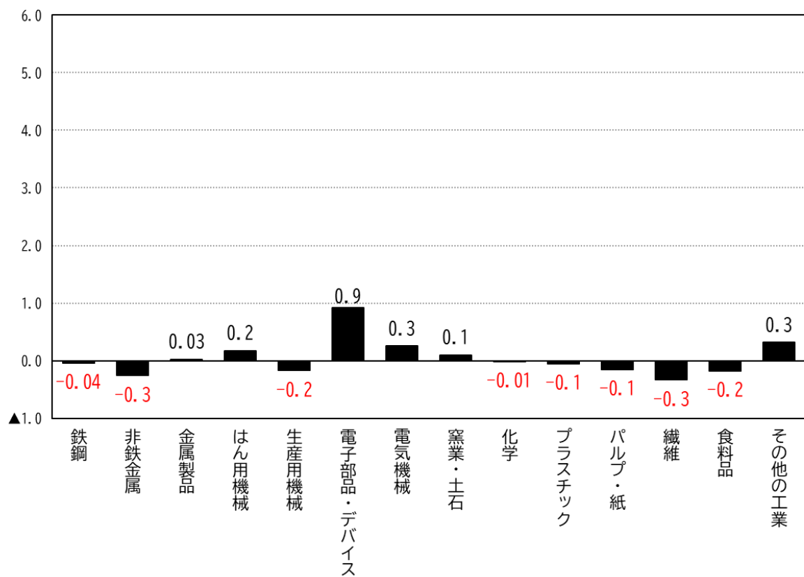
図2 業種別寄与度
