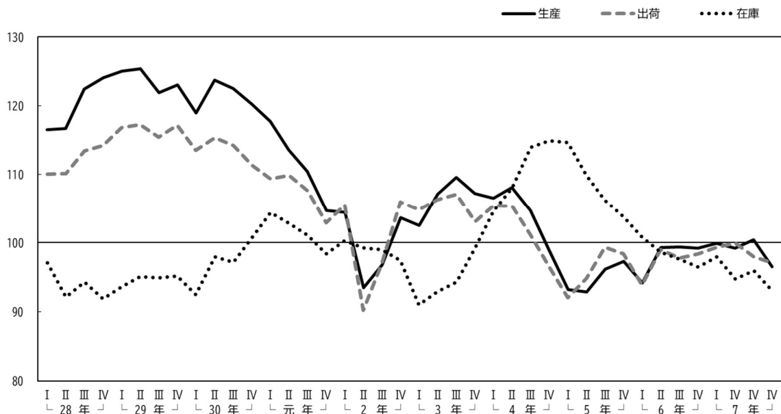
図1 鉱工業指数の四半期別推移
