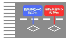
【横断歩道予告標示 (ダイヤマーク)】
